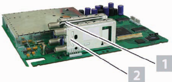
Bild 1: Steckkarte X-DVB-S/PAL duo
