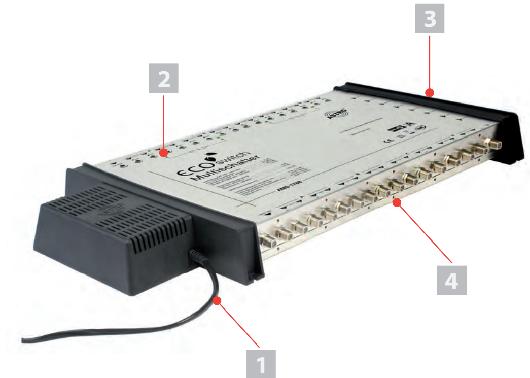
Bild 1: AMS ECOswitch Multischalter (Typ 1788)
