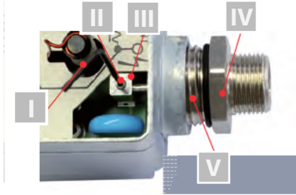
Bild 3: Eingangs- und Ausgangsbuchse montieren
