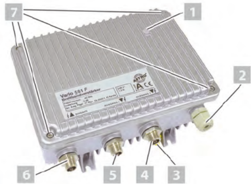
Bild 1: Verstärker VARIO 561 F PG11
