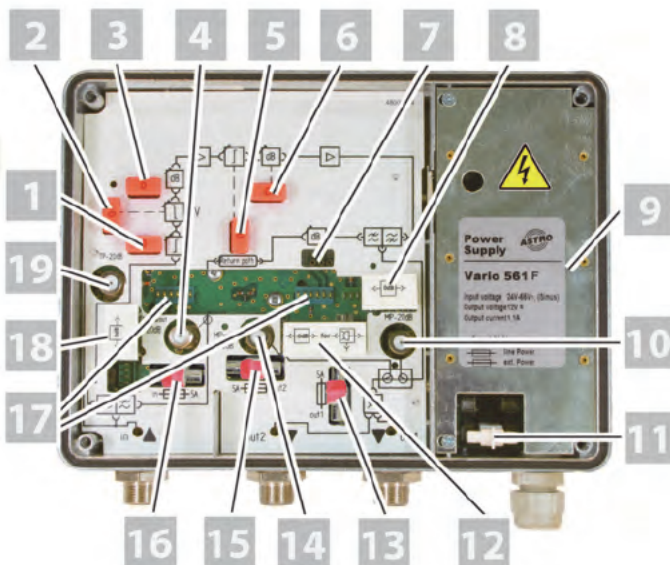
Bild 2: Verstärker VARIO 561 F PG11, innen
