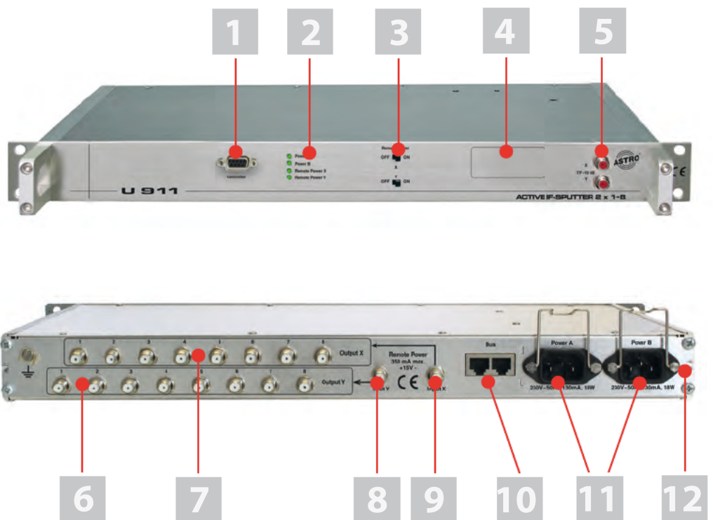
Bild 1: U 911 SAT-Verteilerfeld
