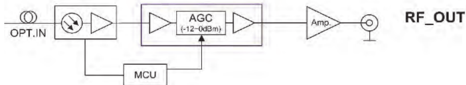
Blockschaltbild MFN-O
