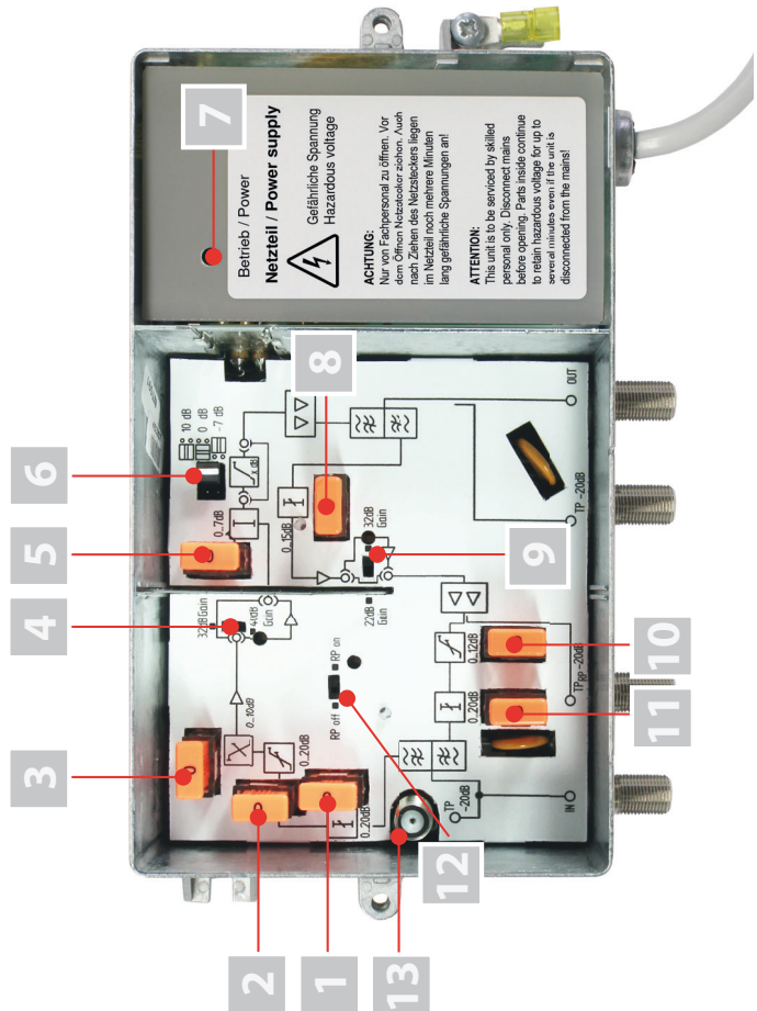
Bild 2: Verstärker HVO V40 P, Innenansicht
