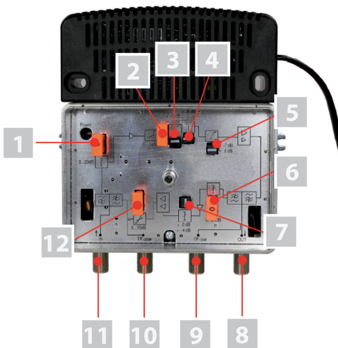
Bild 2: Verstärker HV 426, Innenansicht (HV 436, HV 442 und HV 446 ähnlich)
