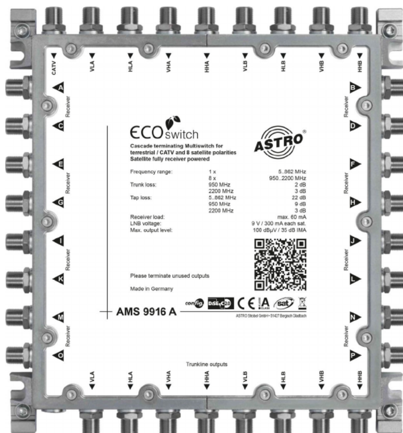
Bild 1: AMS 99.. A Multischalter (Typ 9916 A)
