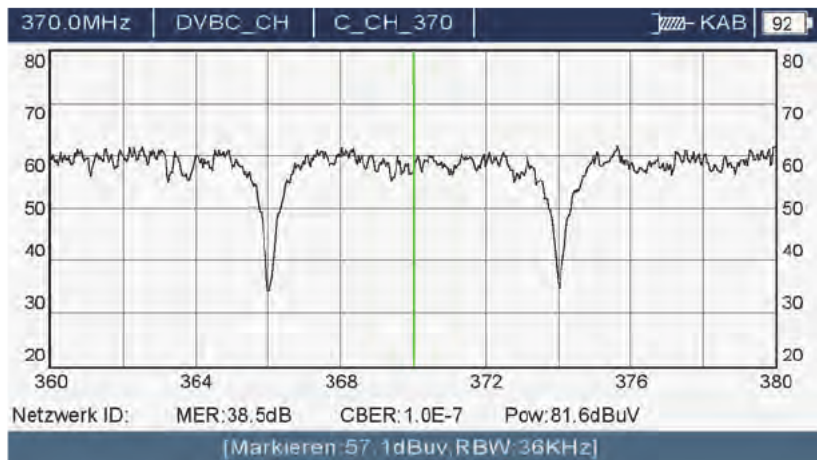
Bild 51: Span 20 MHz
