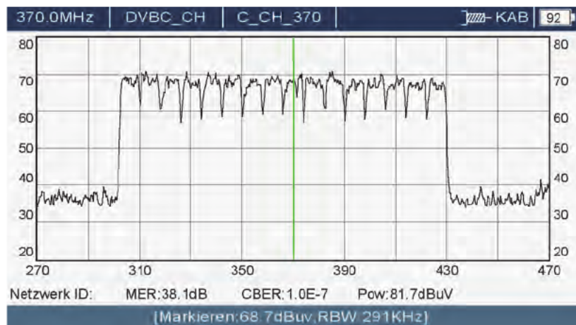
Bild 50: Span 200 MHz
