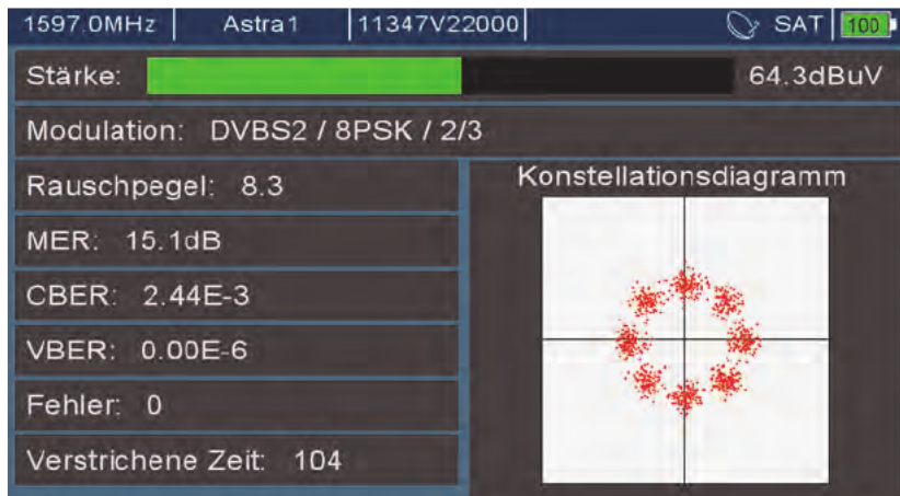
Bild 37: Konstellationsdiagramm
