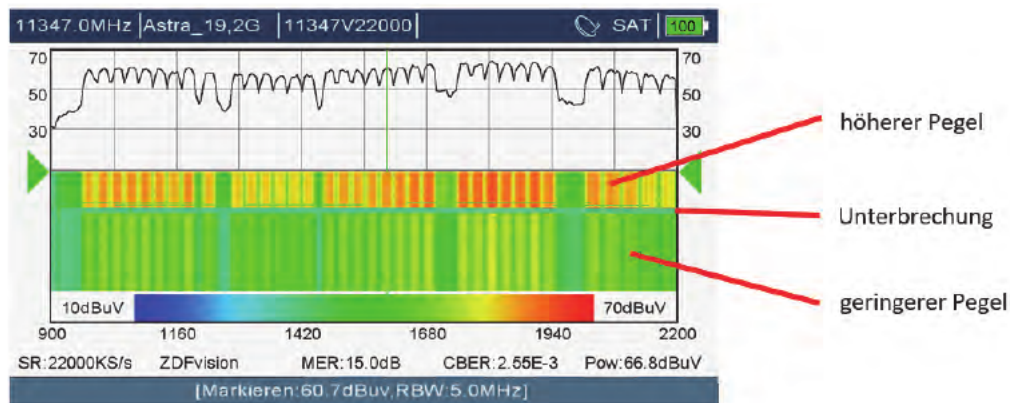
Bild 44: Spektrogramm Modus - unterschiedliche Pegel
