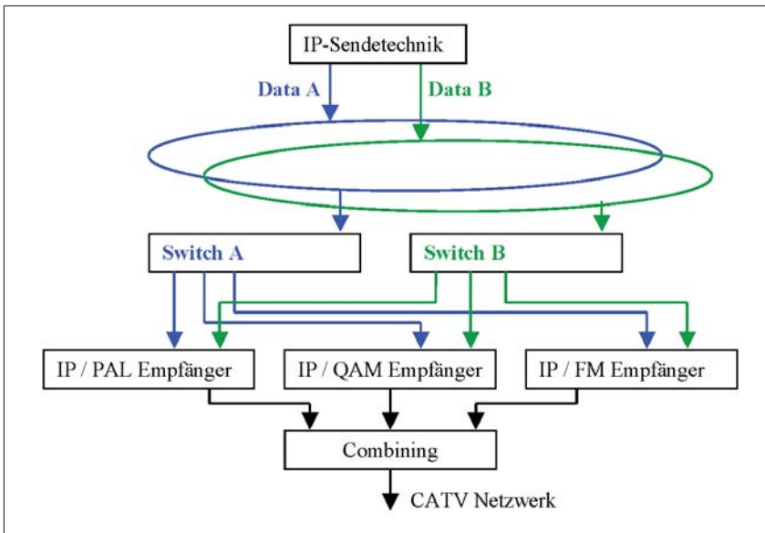
Bild 3: Prinzipschaltbild IP in CATV Signalumsetzung
